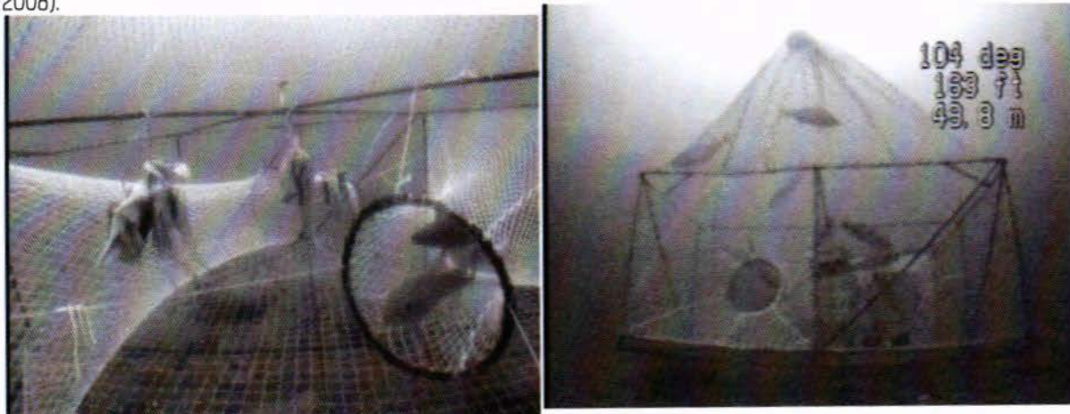
Bilde 4 Undervannsoptak av teina fra Newfoundland, vi ser fisk som går inn og fisk som trekker opp i den flytende takkonstruksjonen.
